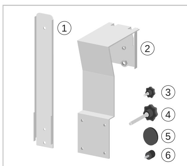
Abb. 2: Lieferumfang
